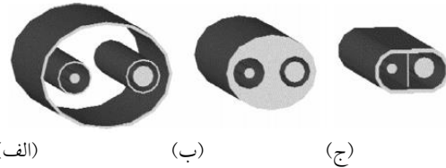
شکل ۱. طرح‌واره‌ای از کاواک‌های (الف): بیضوی، (ب): بازتابنده پخشی و (ج): بازتابنده جفتیده نزدیک [۲۴].
