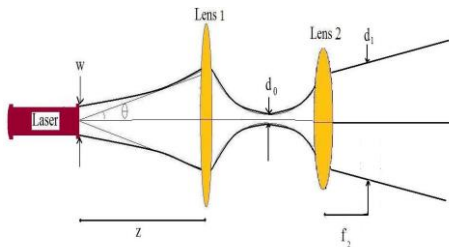
شکل ۷. چیدمانی آزمایشگاهی محاسبه عامل کیفیت پرتو M^2 لیزر (Nd:YAG، عدسی اول، lens 1؛ عدسی دوم، lens 2) [۲۳].
