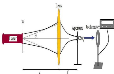
شکل ۶. چیدمان آزمایشگاهی برای اندازه گیری زاویه واگرایی پرتو (1) laser: لیزر Nd:YAG، عدسی، Aperture: روزنه و Joulemeter: ژول متر [۲۶].
