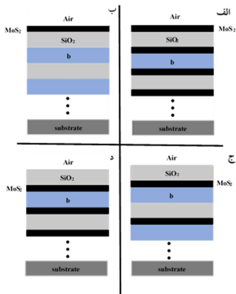
شکل 2 ساختارهای بلورهای فوتونی مورد مطالعه همراه با \text{MoS}_2 (الف) (\text{MoS}_2/\text{SiO}_2/\text{MoS}_2/\text{b})^N (ب) (\text{SiO}_2/\text{b})^N (ج) برای L=1 و L=10 که L تعداد تک‌لایه \text{MoS}_2 می‌باشد، (د) (\text{SiO}_2/\text{MoS}_2/\text{b}/\text{MoS}_2)^N .
