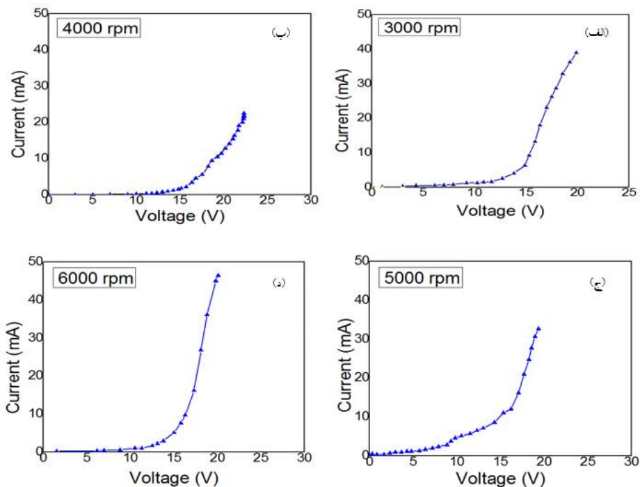
شکل 6. نمودار ولتاژ-جریان برای دیود دولایه با ساختار ITO/PEDOT:PSS/MEH-PPV/ Al(165 nm) با دورها و ضخامت‌های متفاوت برای لایه MEH-PPV
