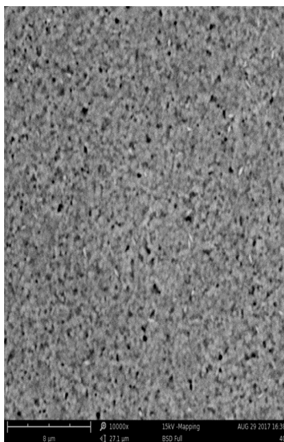
شکل 6: تصویر SEM از پروسکایت حاوی کاتیون Cs. طول مقیاس روی تصویر 8 میکرون می باشد.
