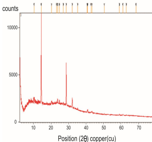
شکل 4. الگوی پراش (XRD) مربوط به پروسکایت حاوی کاتیون Cs.
