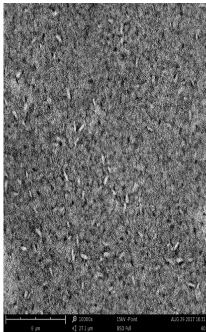
شکل 5. تصویر SEM از پروسکایت حاوی کاتیون RbCs طول مقیاس روی تصویر 8 میکرون می باشد.
