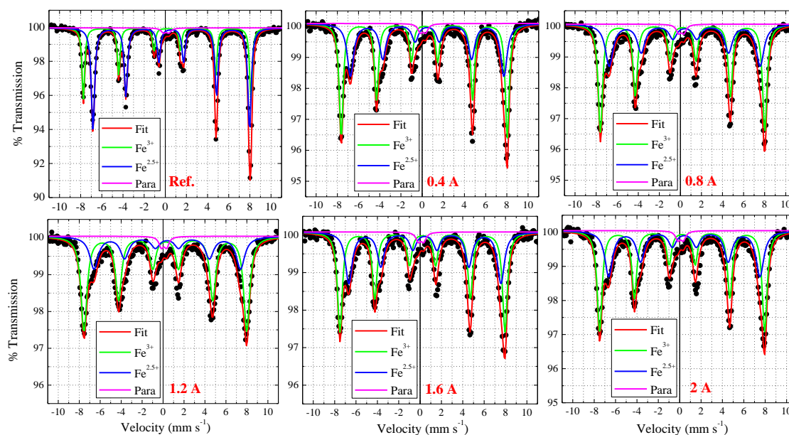
شکل ۵. طیف‌های تجربی و برازش شده موسبائر نمونه شاهد و نانوذرات ساخته شده در این تحقیق، در دمای اتاق.
