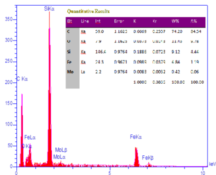
شکل ۵. آنالیز EDX نانولوله‌های رشد یافته بر زیرلایه سیلیکونی.
