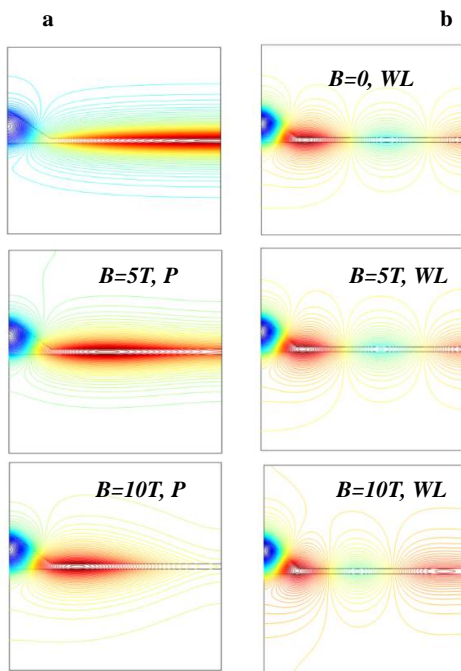
شکل 6. نمای دوبعدی از تابع پوش الکترون در حالت برانگیخته (ستون a)، در حالت برانگیخته دوم (ستون b)، به ازای میدان‌های مغناطیسی مختلف.
