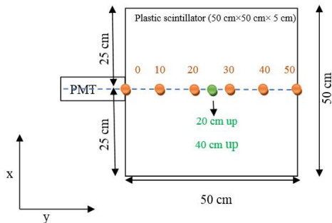
شکل 1. سوسوزن پلاستیک NE102 با ابعاد 50\text{cm} \times 50\text{cm} \times 5\text{cm} که در معرض چشمه ^{137}\text{Cs} با موقعیت‌های مختلف ^{137}\text{Cs} قرار گرفته است.
