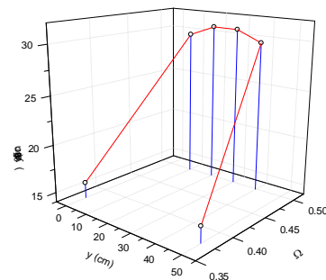
شکل 5. تغییرات بازدهی محاسبه شده، سوسوزن برحسب موقعیت نسبی چشمه-سوسوزن و زاویه فضایی برای سوسوزن پلاستیک NE102، با ابعاد 50\text{cm} \times 50\text{cm} \times 5\text{cm} که در معرض چشمه ^{137}\text{Cs} قرار گرفته است.
