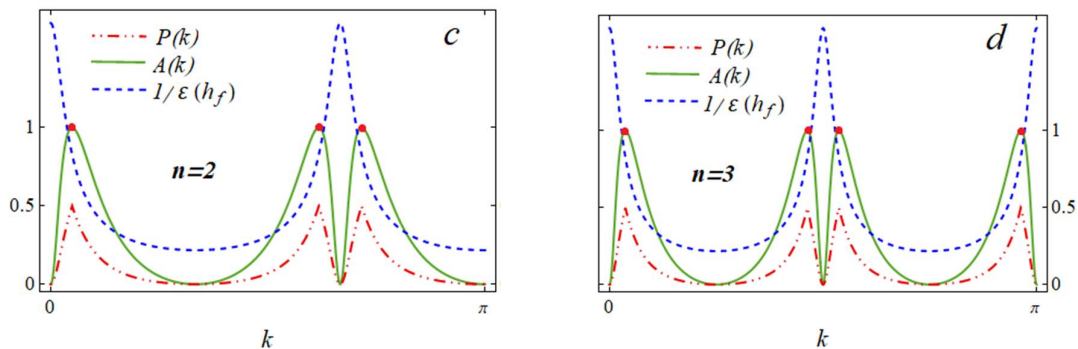
شکل 2. مقایسه بین P(k) ، A(k) و 1/\varepsilon_k^{(n)}(h_f) در حالتی که میدان‌های اولیه و نهایی در دو فاز تعادلی یکسان ( a و b ) و مختلف ( c و d ) هستند. دایره‌های توپر روی نمودار A^{(n)} نشانگر تعداد مدهایی است که شرط گذار فاز دینامیکی را برآورده می‌کند.
