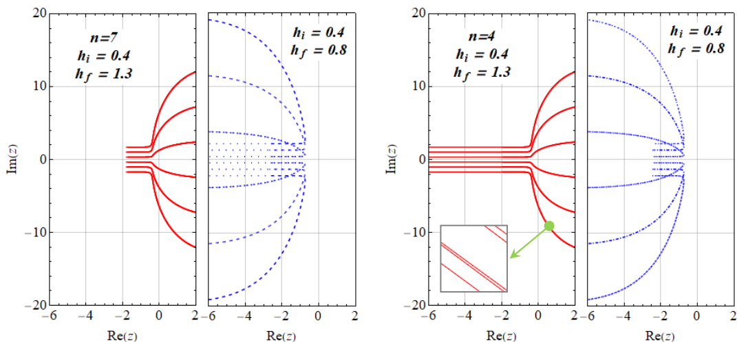
شکل 1. نمودارهای صفرهای فیشر برای مدل خوشه‌ای، n=4 (دو نمودار سمت راست) و n=7 (دو نمودار سمت چپ) در دو حالت دگرگونی ناگهانی در فاز یکسان (خط چین) و در دو فاز مختلف (خط). نمودارها برای پنج مقدار مختلف m \in \{-3, \dots, 2\} رسم شده است.
