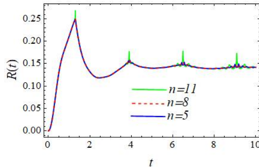
شکل 4. تابع احتمال بازگشت برحسب زمان برای شبکه به بزرگی N=1000 و برای خوشه‌های n=5, 8, 11 در حالتی که میدان‌های اولیه و نهایی در دو فاز تعادلی مختلف هستند.
