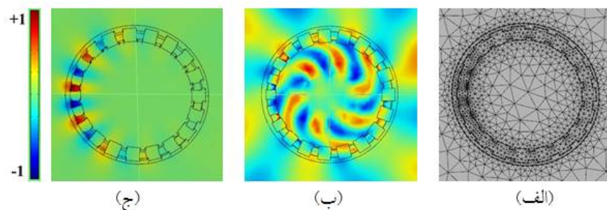
شکل 2. الف: یک مشبک‌سازی نمونه، در نواحی مختلف ساختار برای شبیه‌سازی و بدست آوردن الگوی توزیع مدی در ب و ج. ب: پراکندگی امواج چشمگیر بوده، در حالی که در ج: تمرکز مدی در ناحیه شیاری بین حفره‌های مکعبی هوا در مسیر دایروی پیرامون میکرو دیسک و در سمت چپ آن مشهود است.
