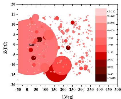
شکل 1. توزیع جرم (برحسب جرم خورشید) و شعاع ستارگان نسبت به صفحه کیهشانی (طول کیهشانی).
