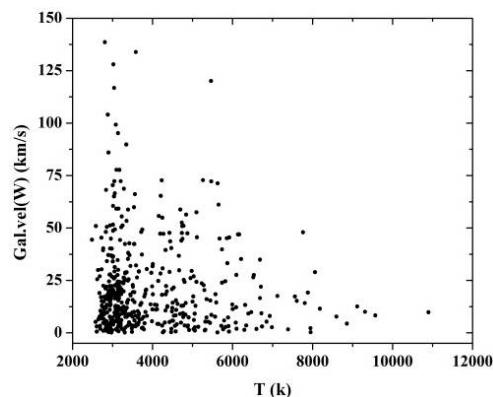
شکل 5 ب. سرعت کهکشانی W بر حسب دمای ستارگان.
