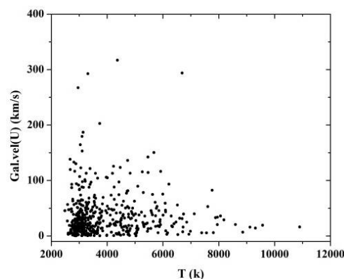
شکل 5 الف. سرعت کهکشانی U بر حسب دمای ستارگان.
