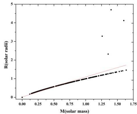
شکل 7. وابستگی شعاع ستاره و جرم آن برای ستارگان سنگین‌تر.
