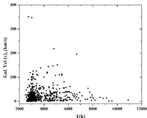
شکل 5 ج. سرعت کهکشانی V بر حسب دمای ستارگان.
