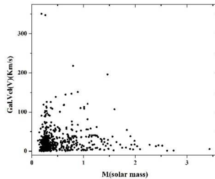
شکل 3 ب. سرعت کهکشانی V برحسب جرم ستارگان.
