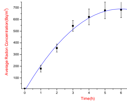
شکل 3. منحنی تغییرات متوسط غلظت رادون در اتاقک اندازه‌گیری برای یک مکان نمونه در کف اتاق و در شرایط بدون تهویه.
